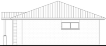
Elevation 4
