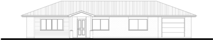
Elevation 1
