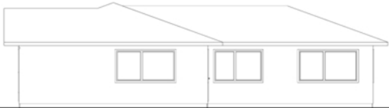
Elevation 3 1:150
