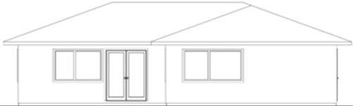
Elevation 2 1:150
