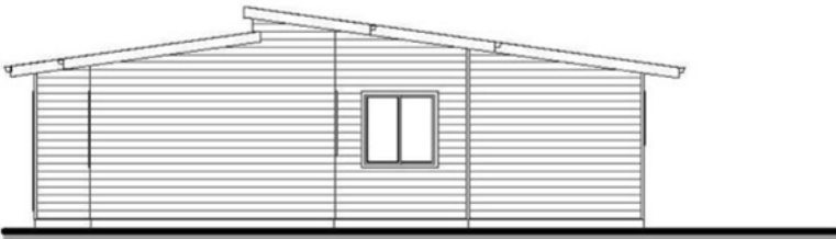
Elevation 4
