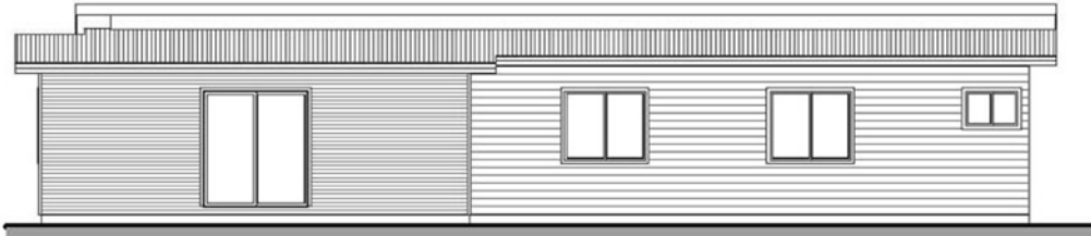
Elevation 1
