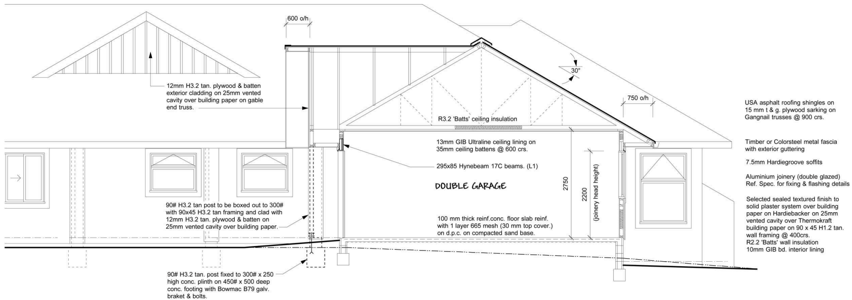
SECTION D-D
